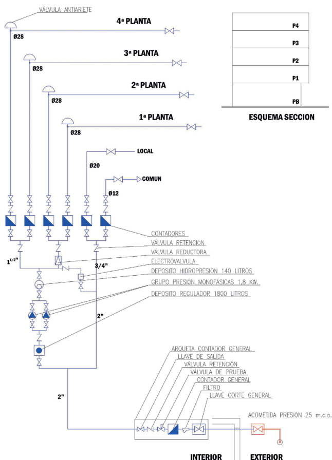
ESQUEMA VERTICAL DE DISTRIBUCIÓN DE AGUA POTABLE EN UN EDIFICIO DE PB + 4P (4viviendas)
