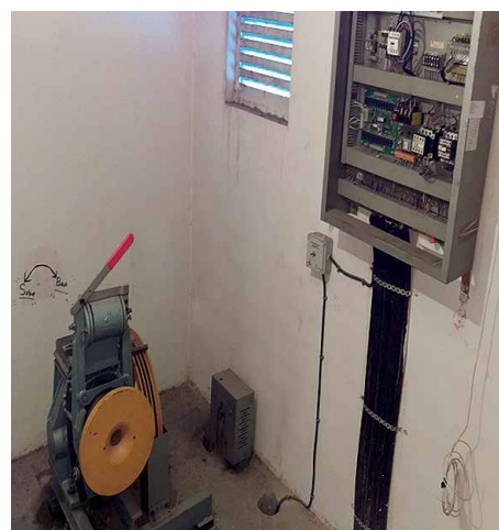
Cuarto o sala de máquinas.
