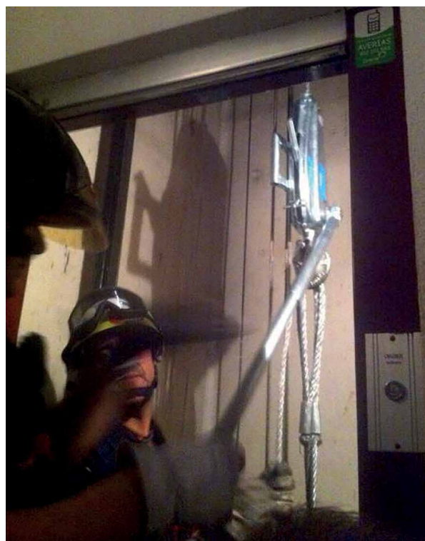
Tracción ascendente mediante tráctel.
